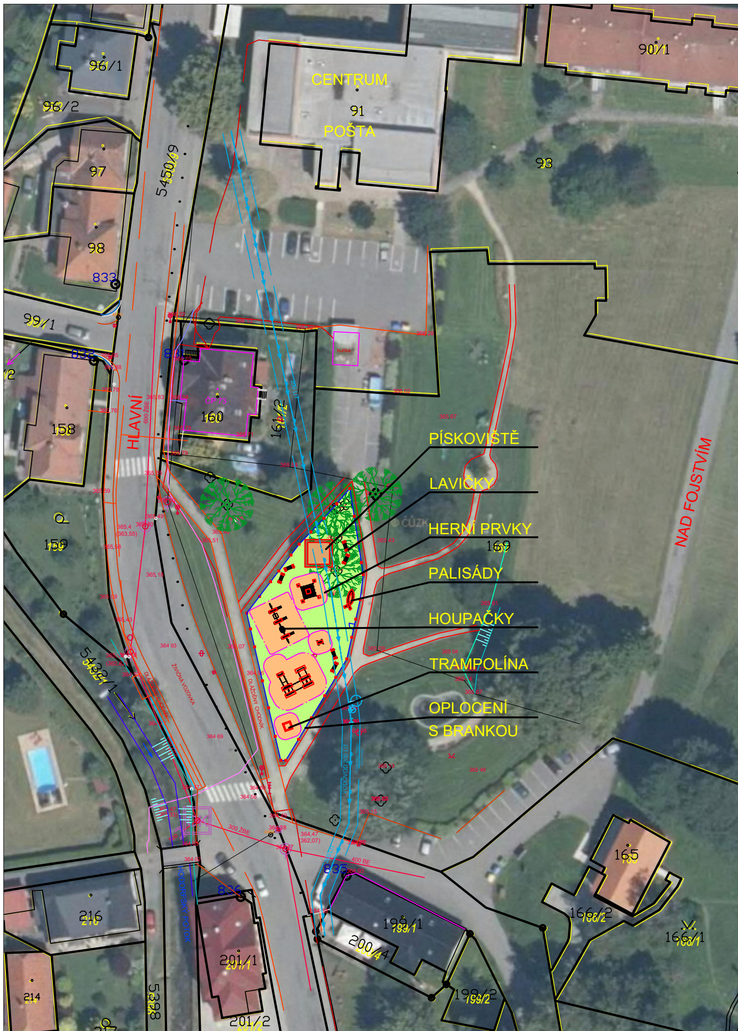
DĚTSKÉ HŘIŠTĚ - OSAZENÍ HERNÍCH PRVKŮ
